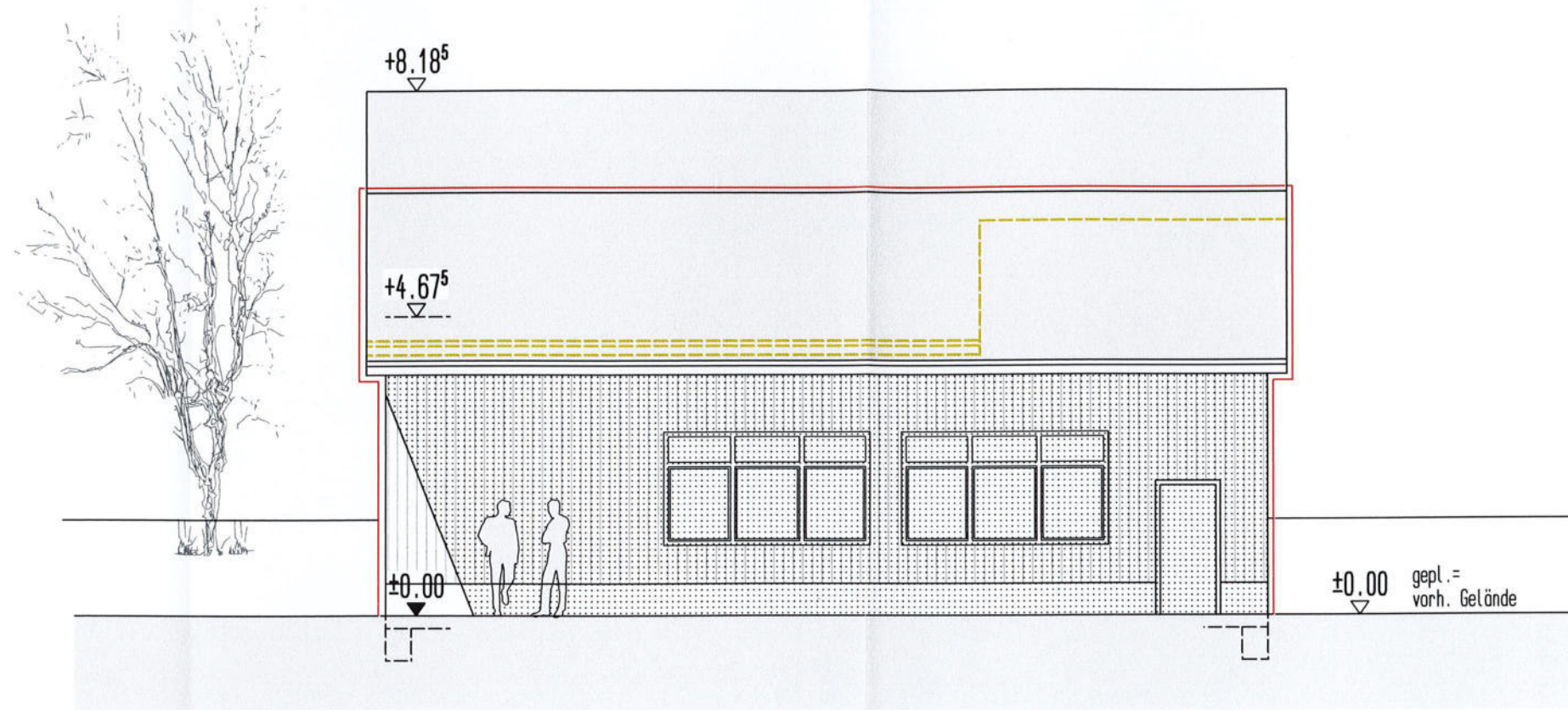
ANSICHT NORD-WEST
