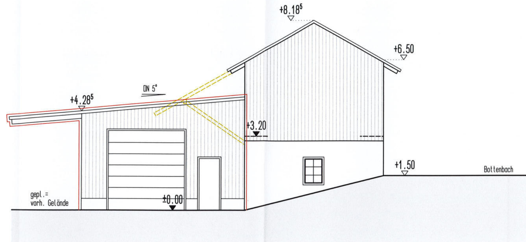
ANSICHT SUD-WEST
