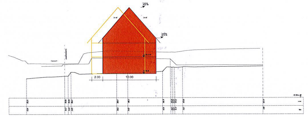
Schnitt
