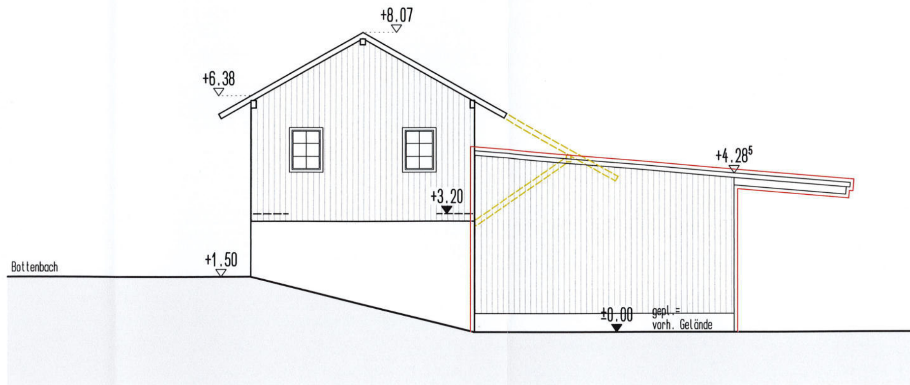
ANSICHT NORD-OST
